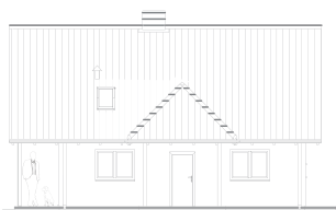
elewacja frontowa
